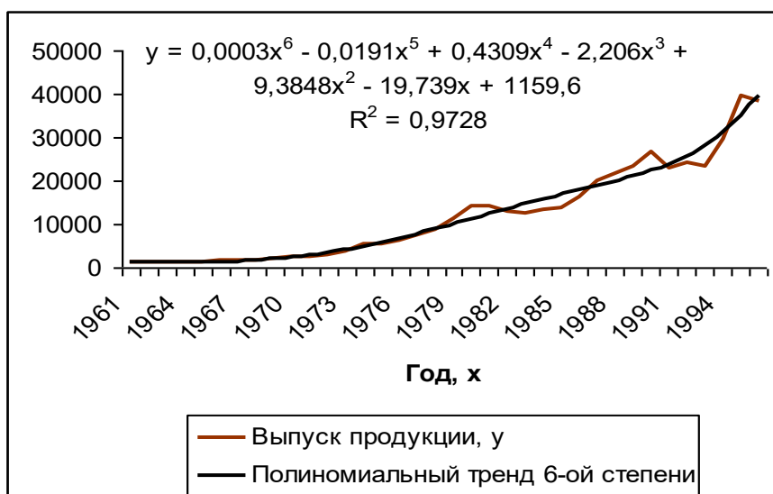
Рис.7. Полиномиальный тренд
