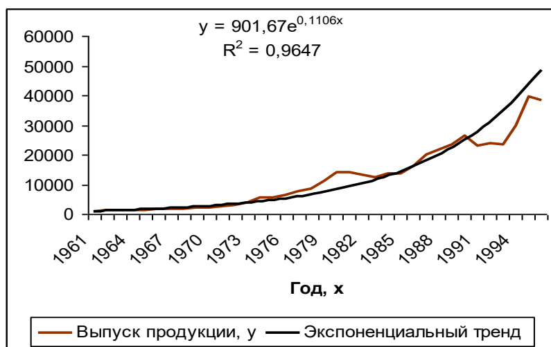
Рис.9. Экспоненциальный тренд
