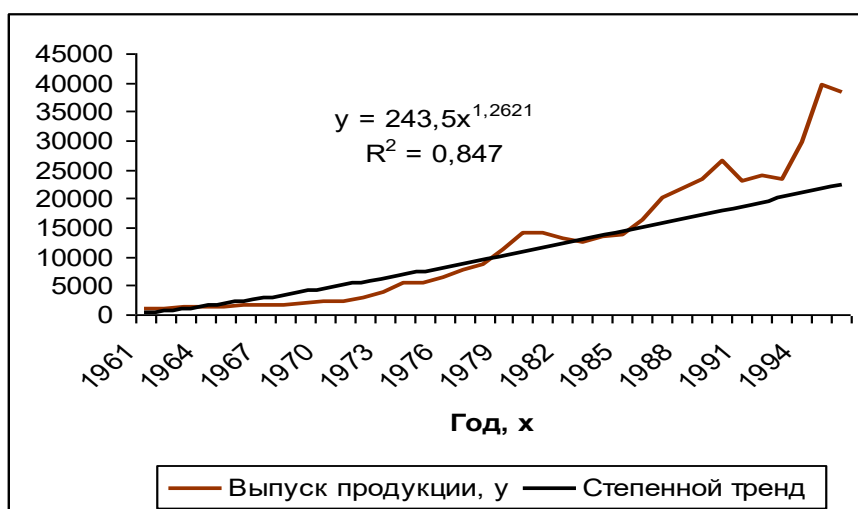
Рис.8. Степенной тренд
