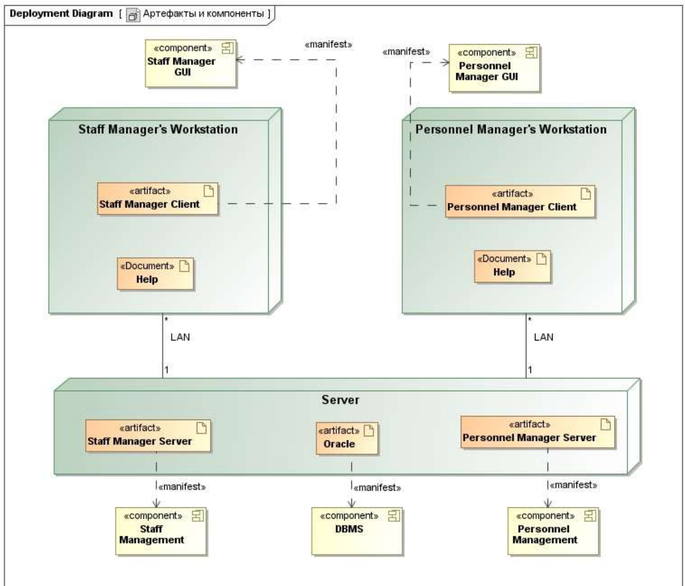
Рисунок 2. Пример UML-диаграммы размещения для информационной системы «Отдел кадров»
