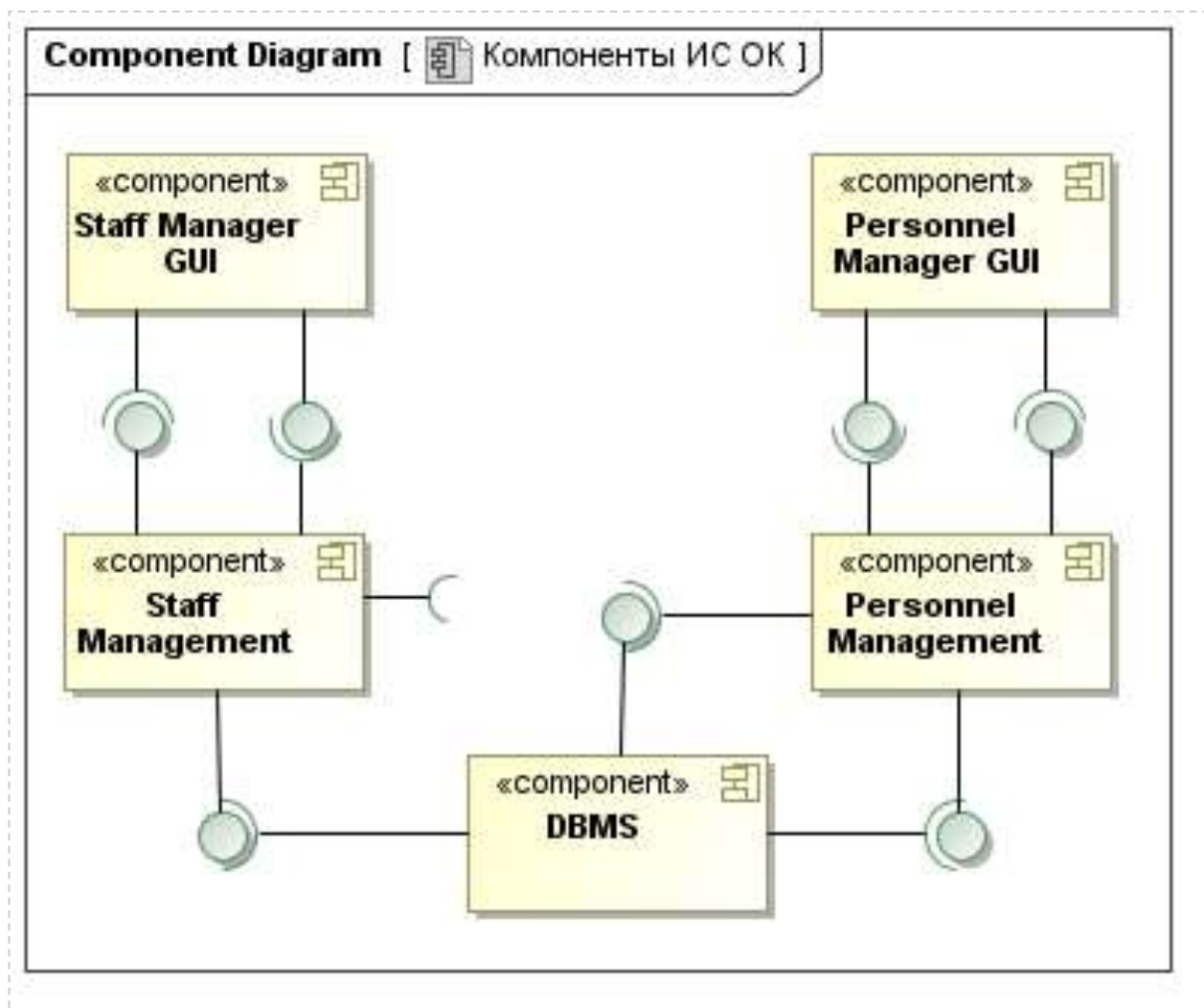
Рисунок 1. Пример UML-диаграммы компонентов для информационной системы «Отдел кадров»
