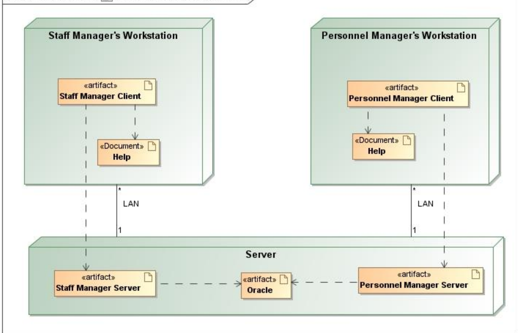
Deployment Diagram [ Зависимости между артефактами ]
